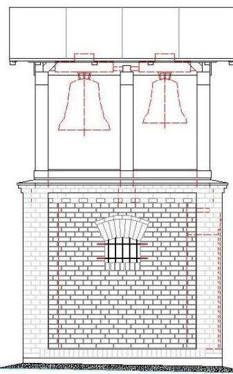
ELEWACJA POŁUDNIOWA
