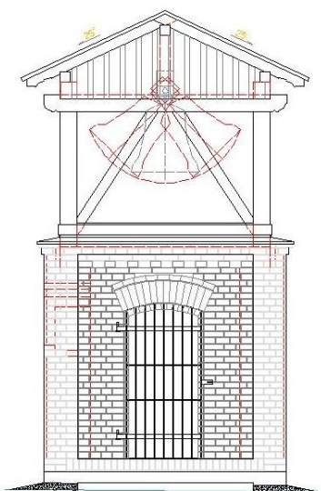
ELEWACJA WSCHODNIA
