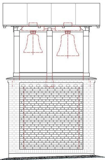
ELEWACJA PÓŁNOCNA
